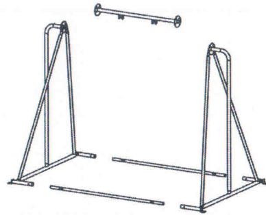
Elements assembling scheme (Общая схема сборки элементов комплекса)
