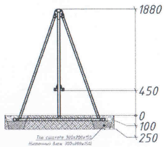
The equipment mounting plan (Схема монтажа оборудования)
